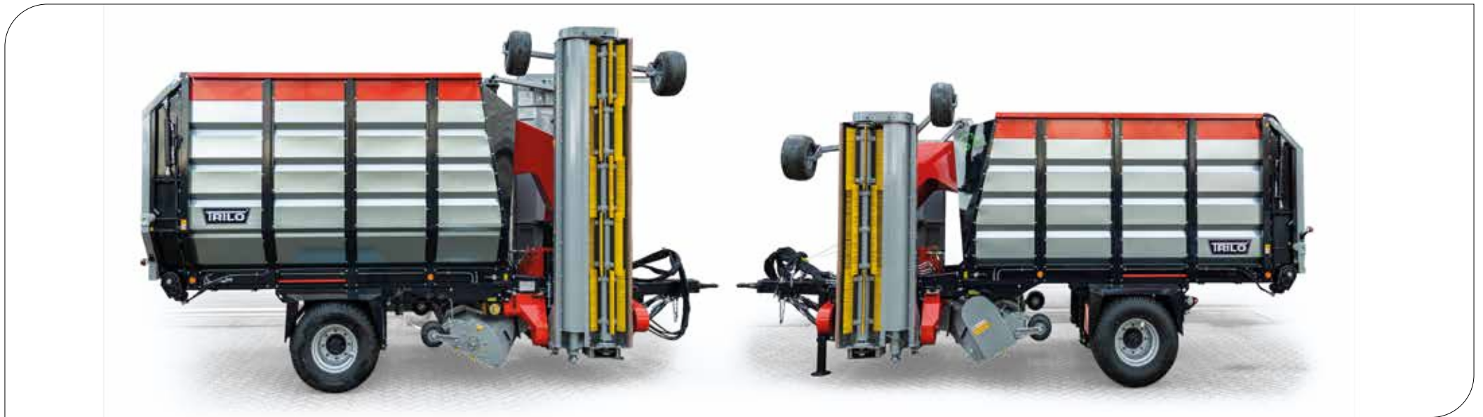
TRILO-Graszuigwagens met vleugels hebben een werkbreedte van 5.8 of 7.6 m.
